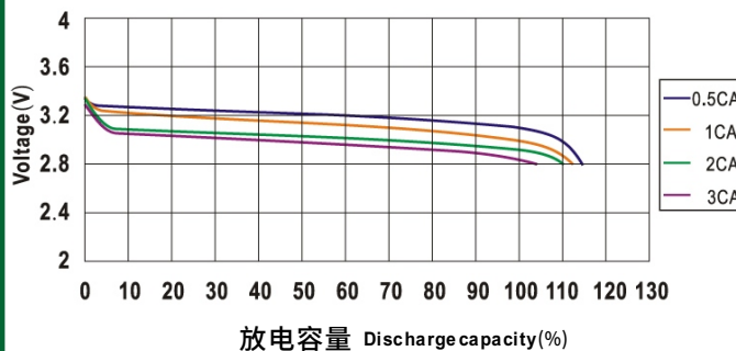
常温下LYP类电池的放电特性曲线
