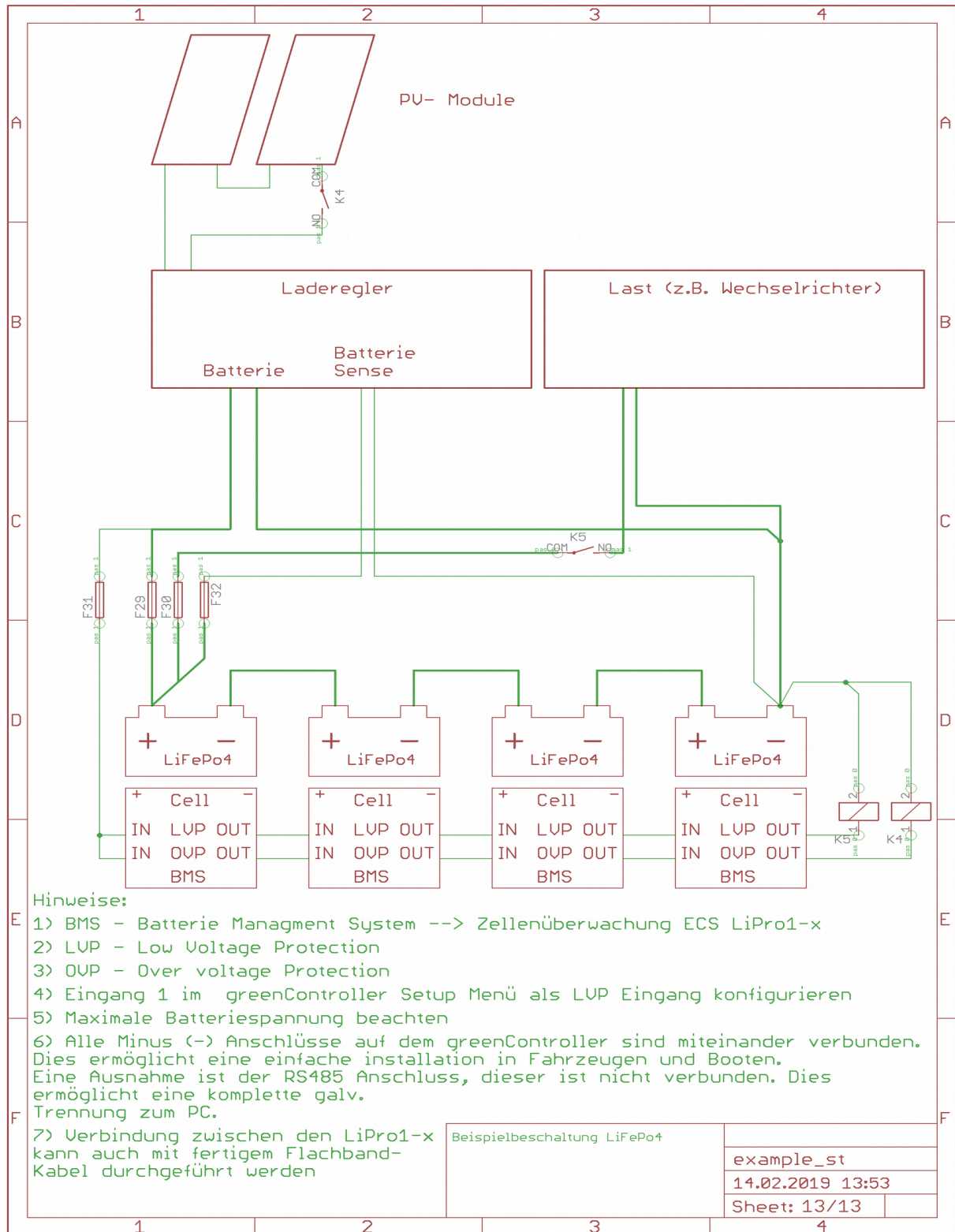
Abbildung 9: Lipro1-x V2 Beispiel – Beliebiger Laderegler
