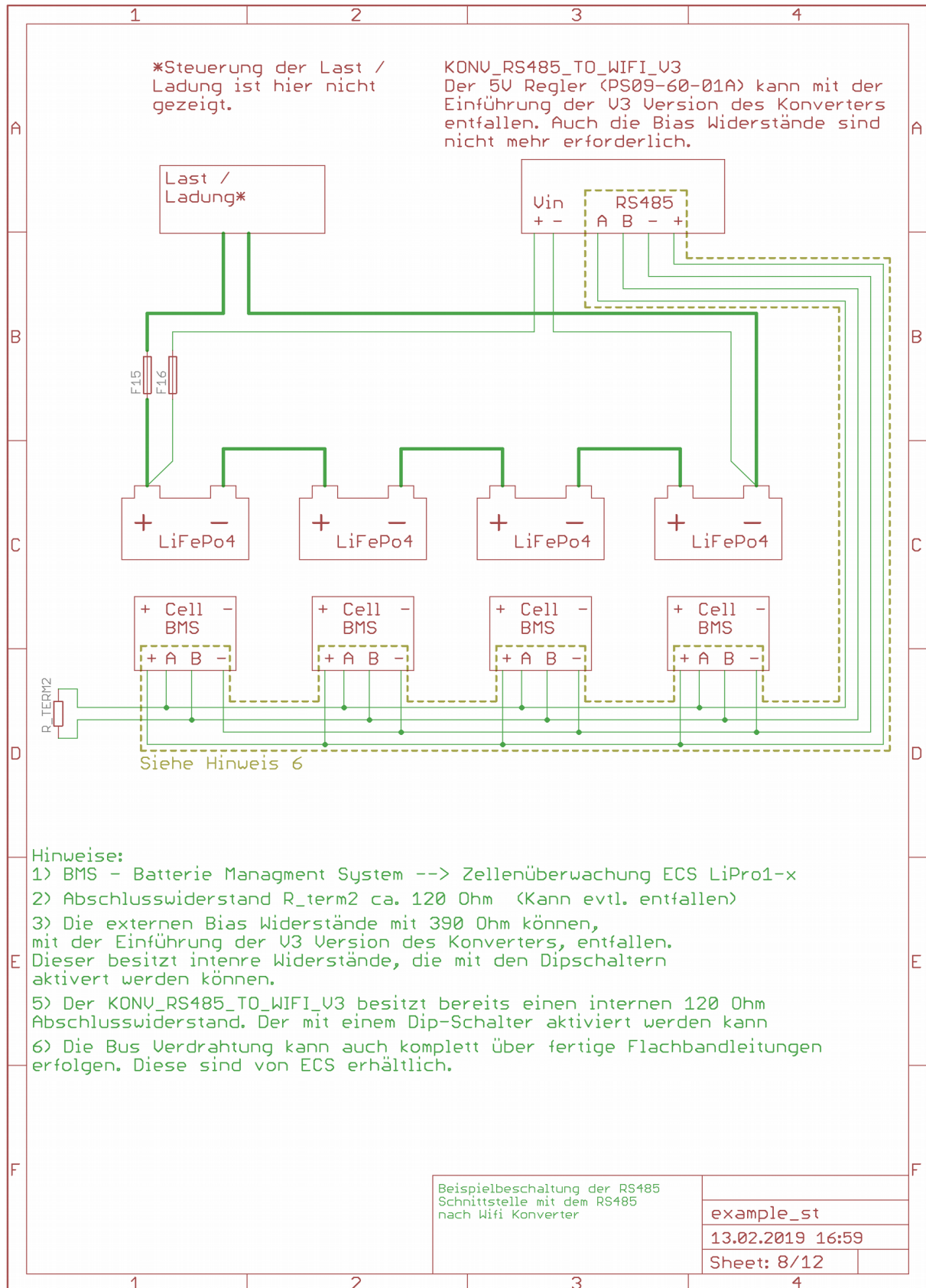
Abbildung 11: LiPro1-x V2 Beispiel – RS485 zum WIFI Konverter
