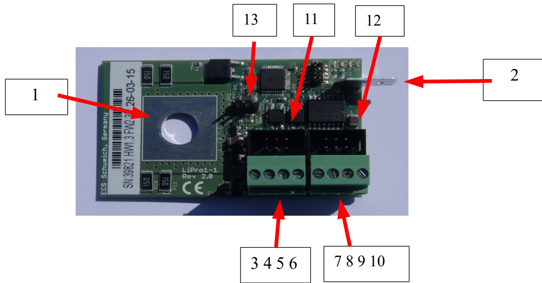
Abbildung 6: LiPro 1-1 V2 – Anschlussbelegung
