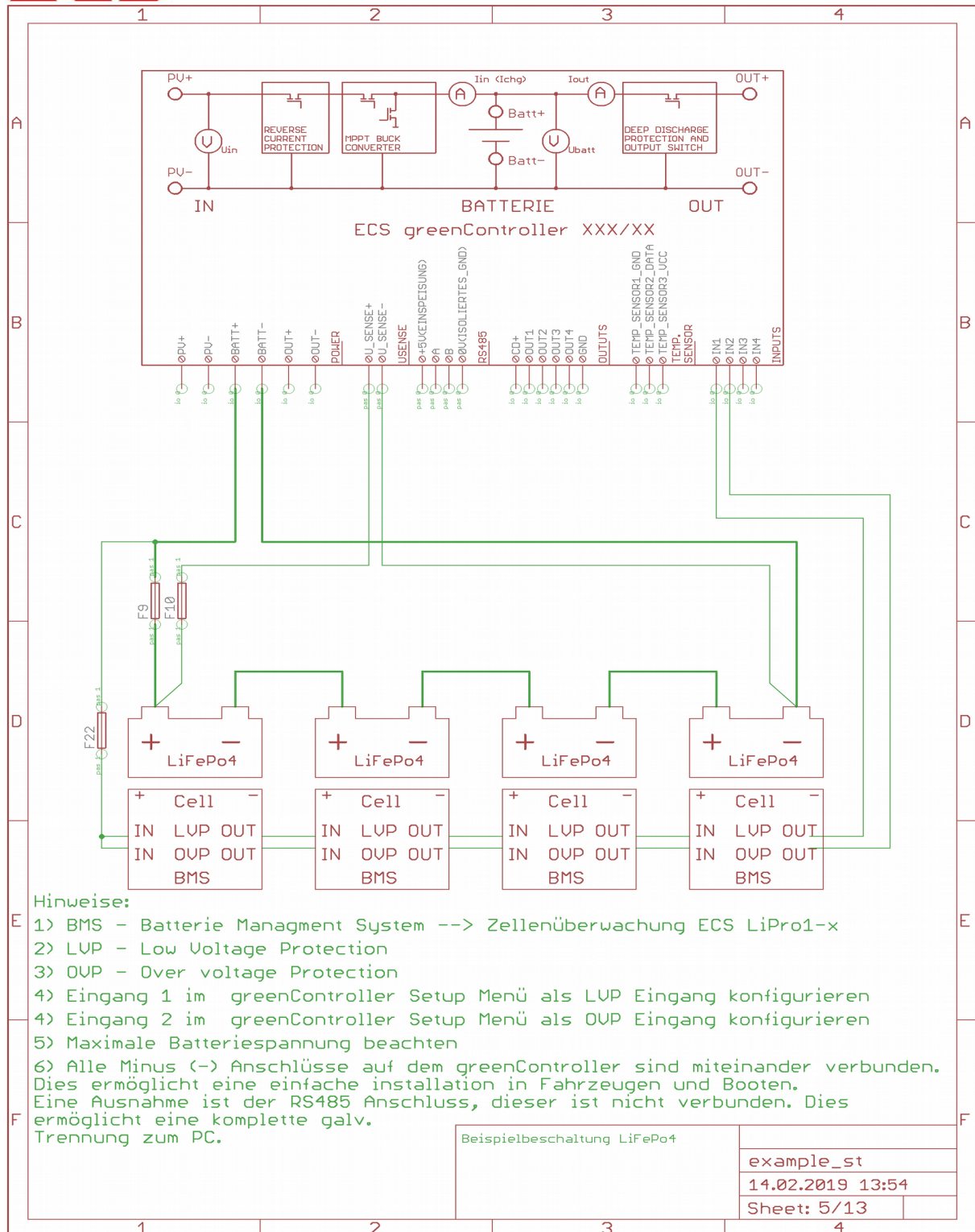
Abbildung 8: LiPro 1-x V2 Beispiel – Digital mit greenController
