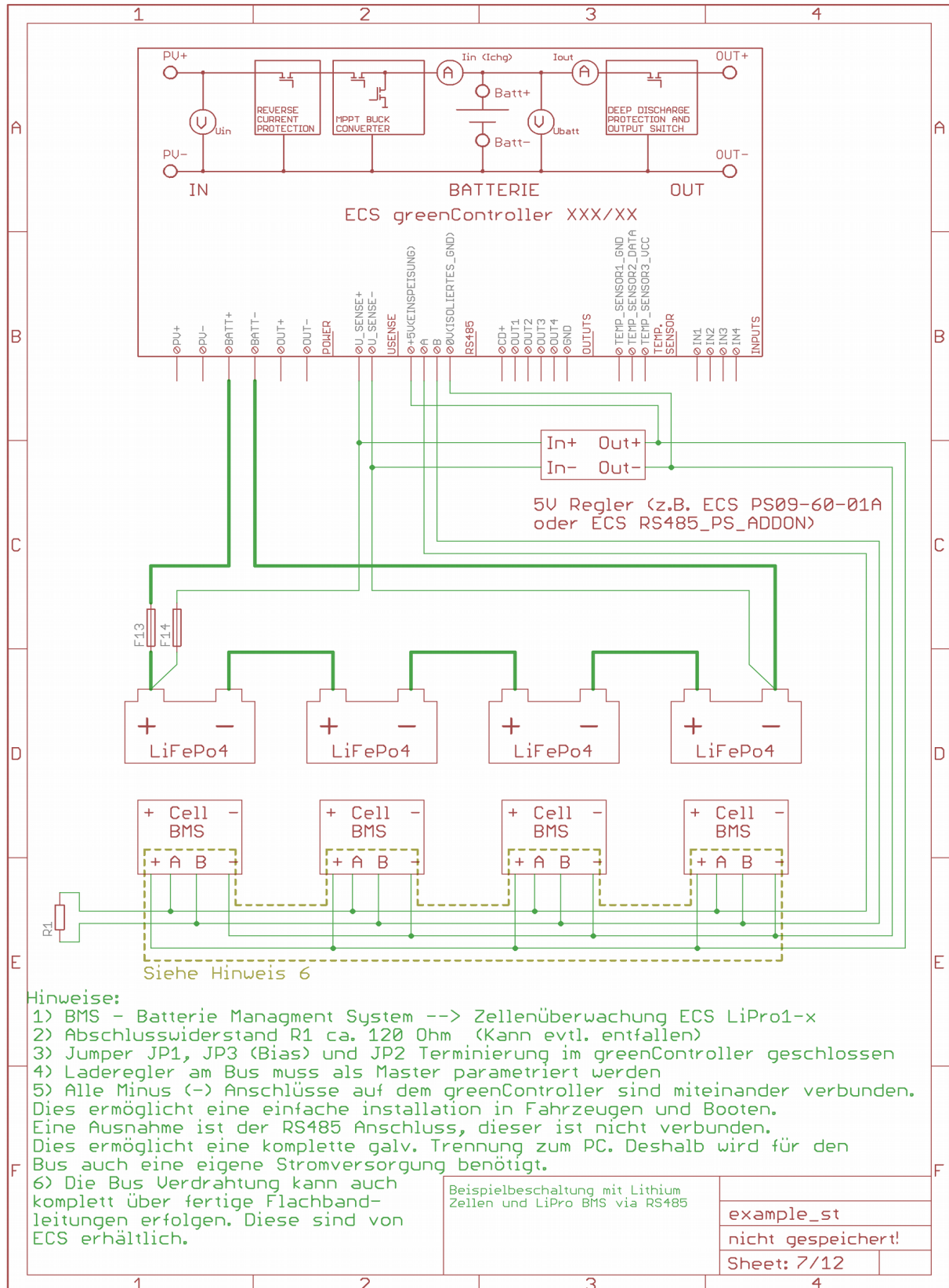
Abbildung 10: LiPro1-x V2 Beispiel – Lithium Zellen, RS485
