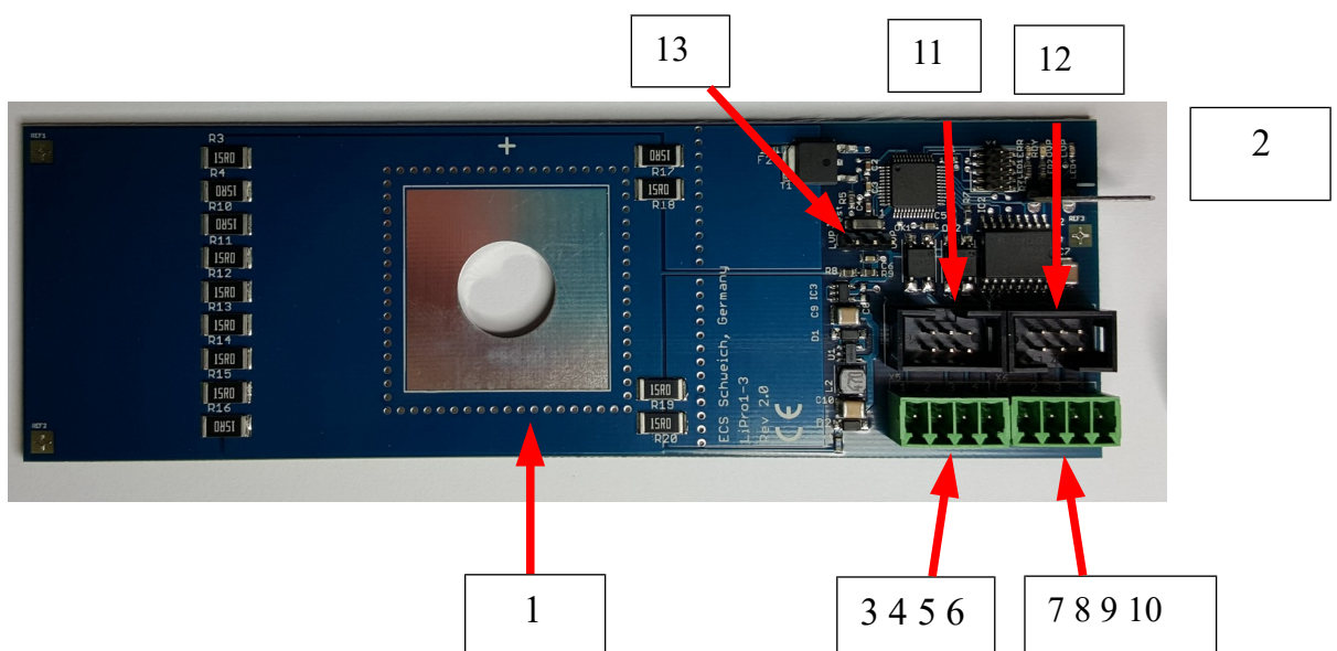
Abbildung 7: LiPro 1-3 V2 – Anschlussbelegung
