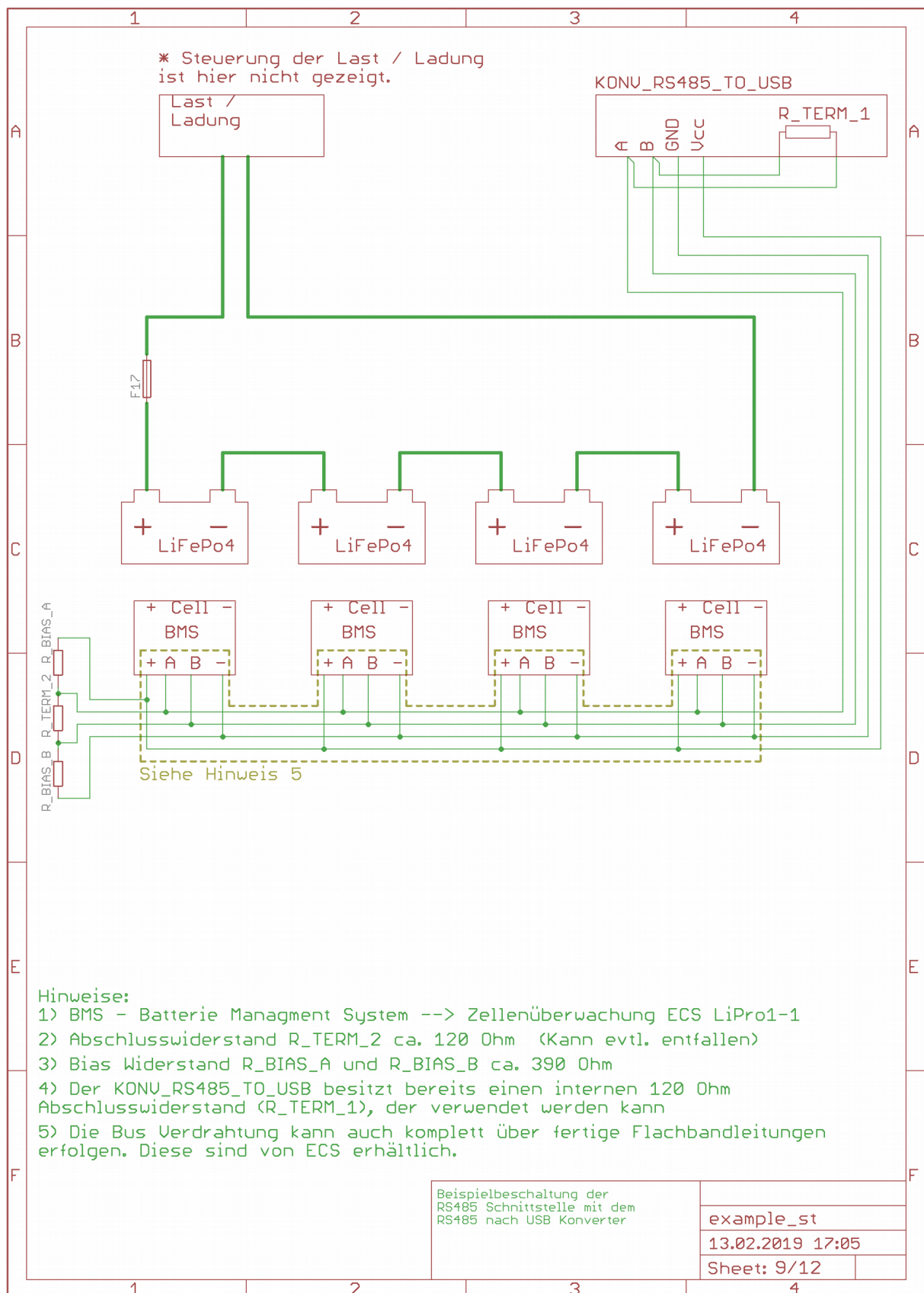
Abbildung 12: Lipro1-x V2 Beispiel – RS485 zum USB Adapter
