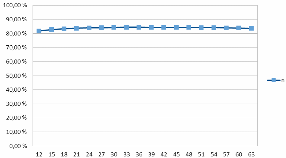
Abbildung 2: Diagramm Wirkungsgrad bei U_{in} 3,0 V
