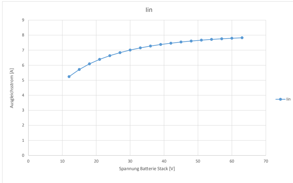
Abbildung 4: Diagramm Ausgleichsstrom Zelle vs. Battery Stack Spannung
