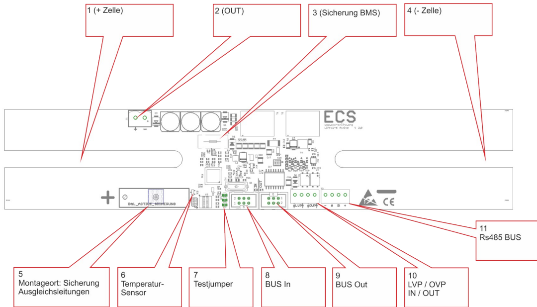
Abbildung 7: Position der Anschlüsse und Komponenten
