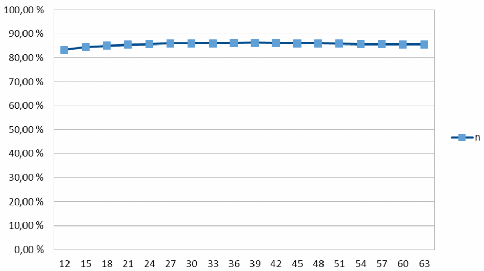
Abbildung 3: Diagramm Wirkungsgrad bei U_{in} 4,0 V
