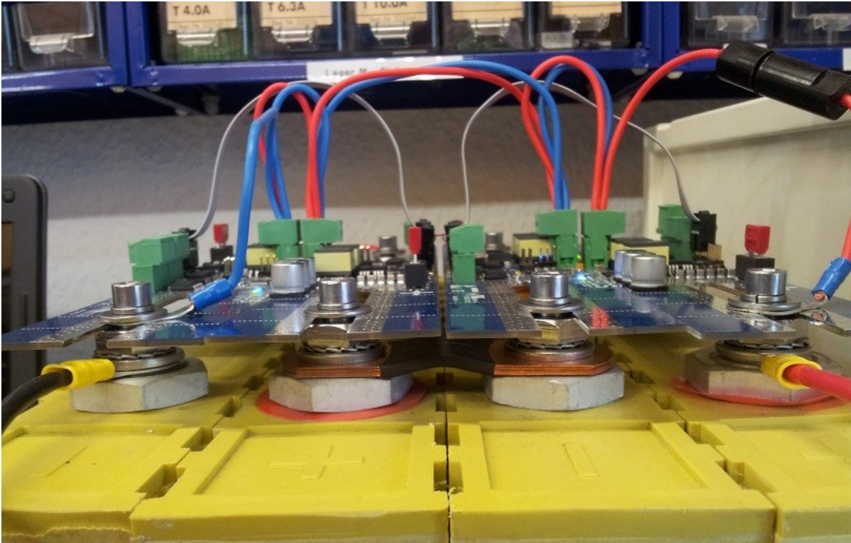
Abbildung 6: Montage (Ansicht von der Seite)
